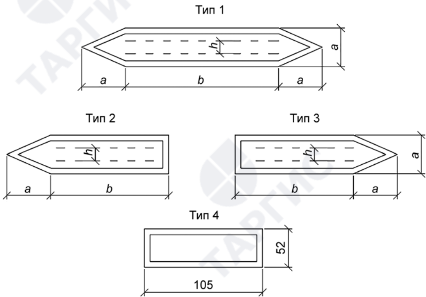
Рисунок 3 — Маркировочные щитки
