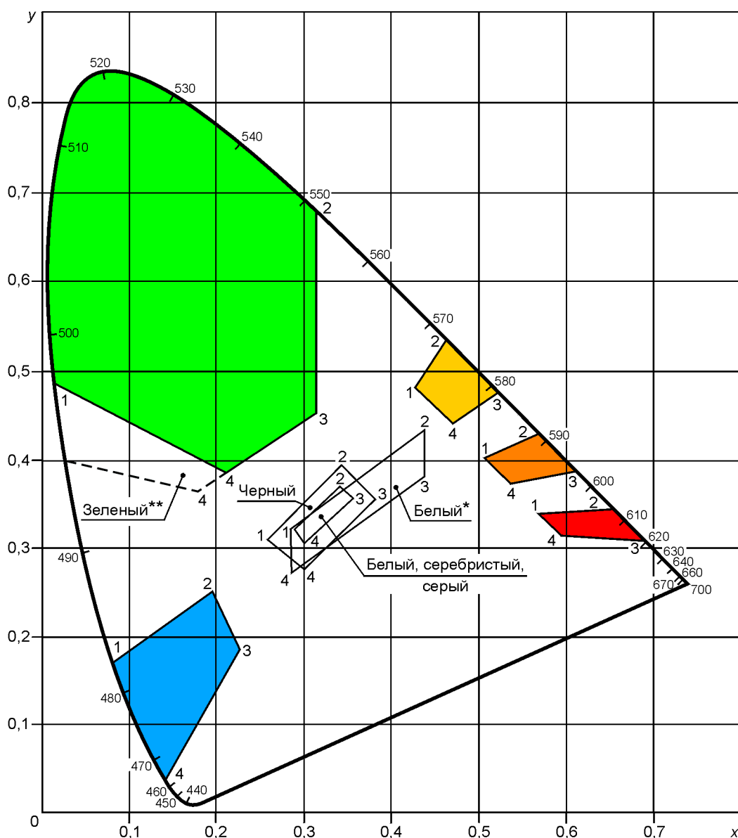
Рисунок 2 — График цветовых областей для знаков с внутренним и внешним освещением
